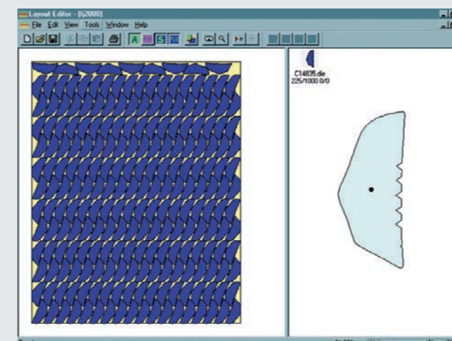
Optimiertes Reihennesting
